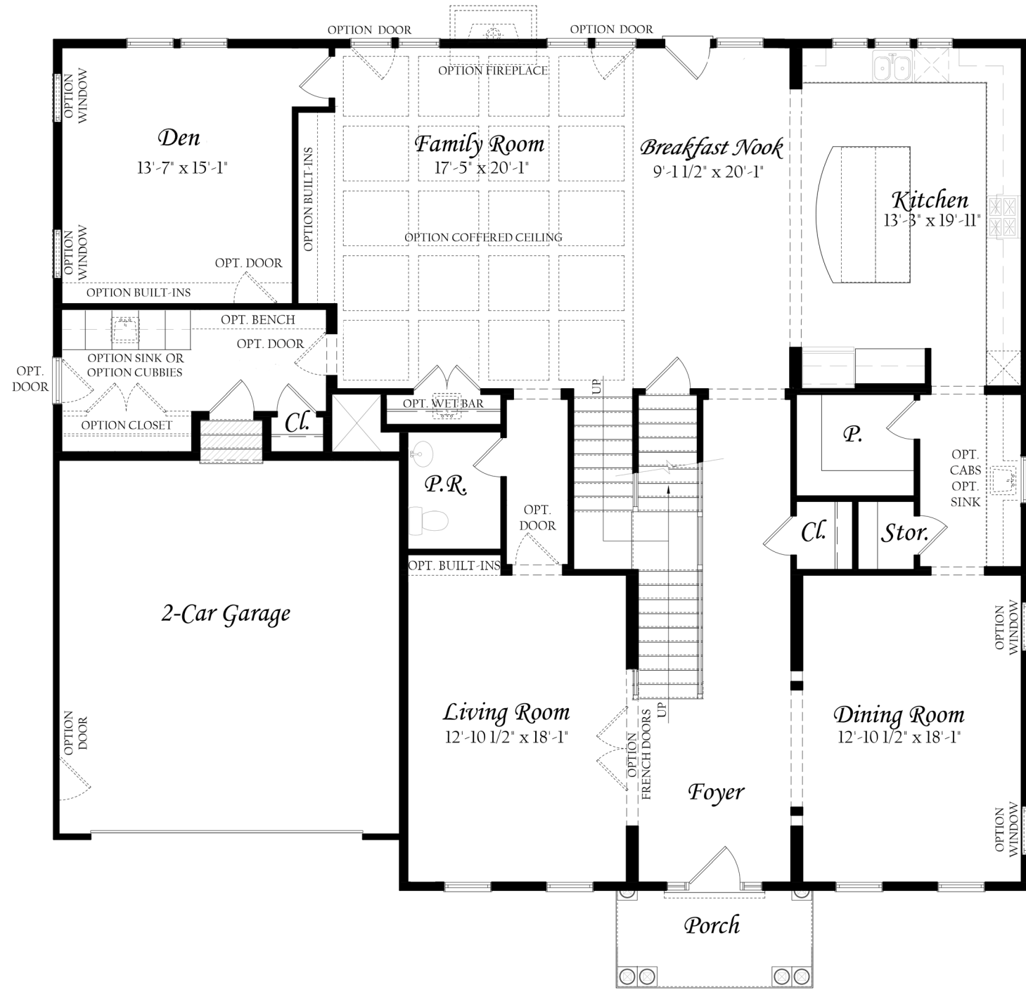
Elevation A
